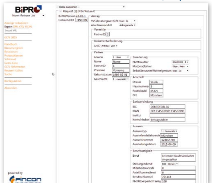
BiPROskop – Struktursicht
