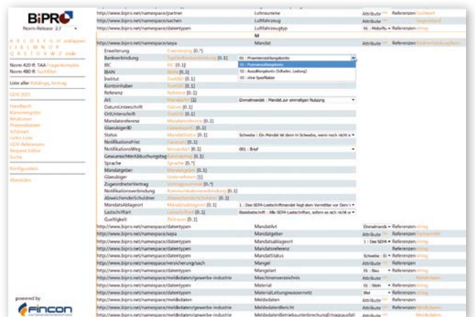
BiPROskop – Objektsicht
